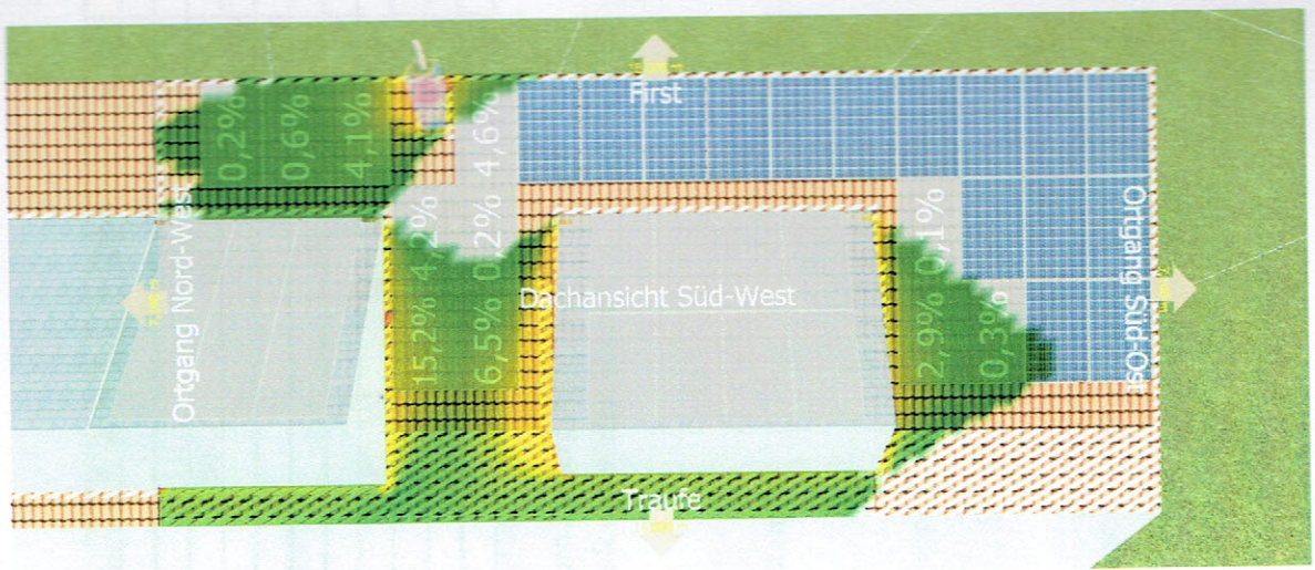
Dach: Schattenhäufigkeitsverteilung
